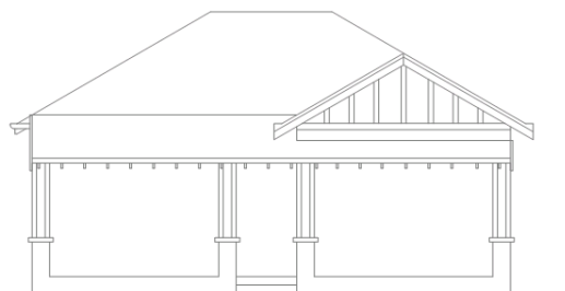
EXISTING ELEVATION 5
