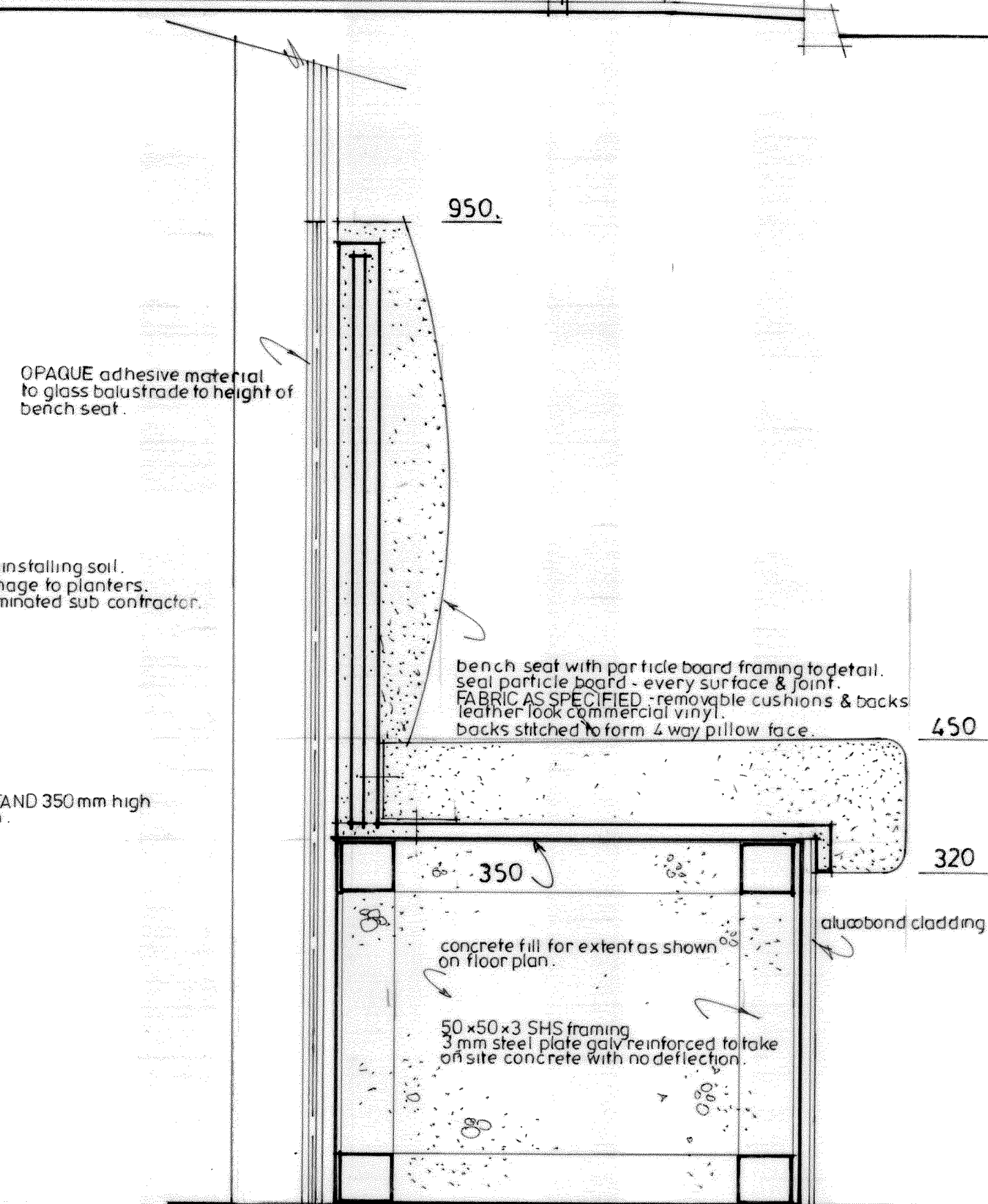
K. SECTION. 3. SCALE 1:20.
