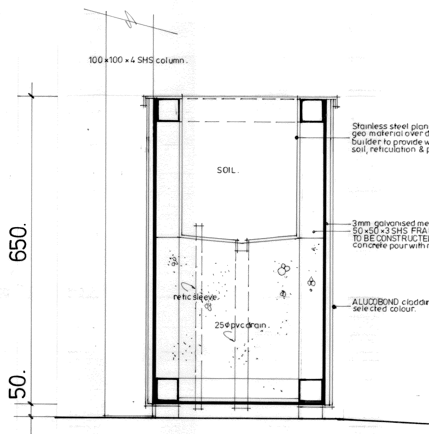
K. SECTION. 3. SCALE 1:20.
