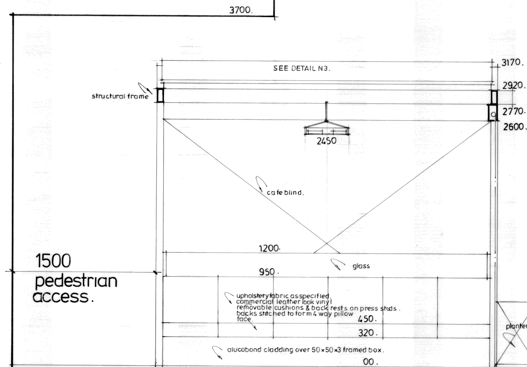
K. SECTION. 3. SCALE 1:20.
